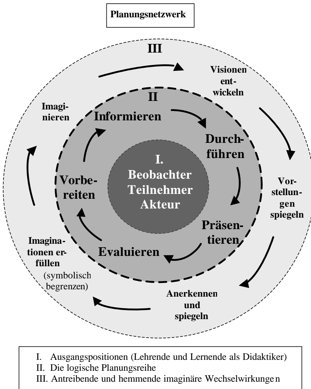
Schaubild 11: Planungsnetzwerk
